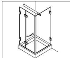
Typ 230 Eckkabine 1 Drehtür am Fixteil 1 Seitenwand
