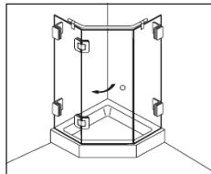
Typ 225 Fünfeckkabine 1 Drehtür | 2 Fixteil
